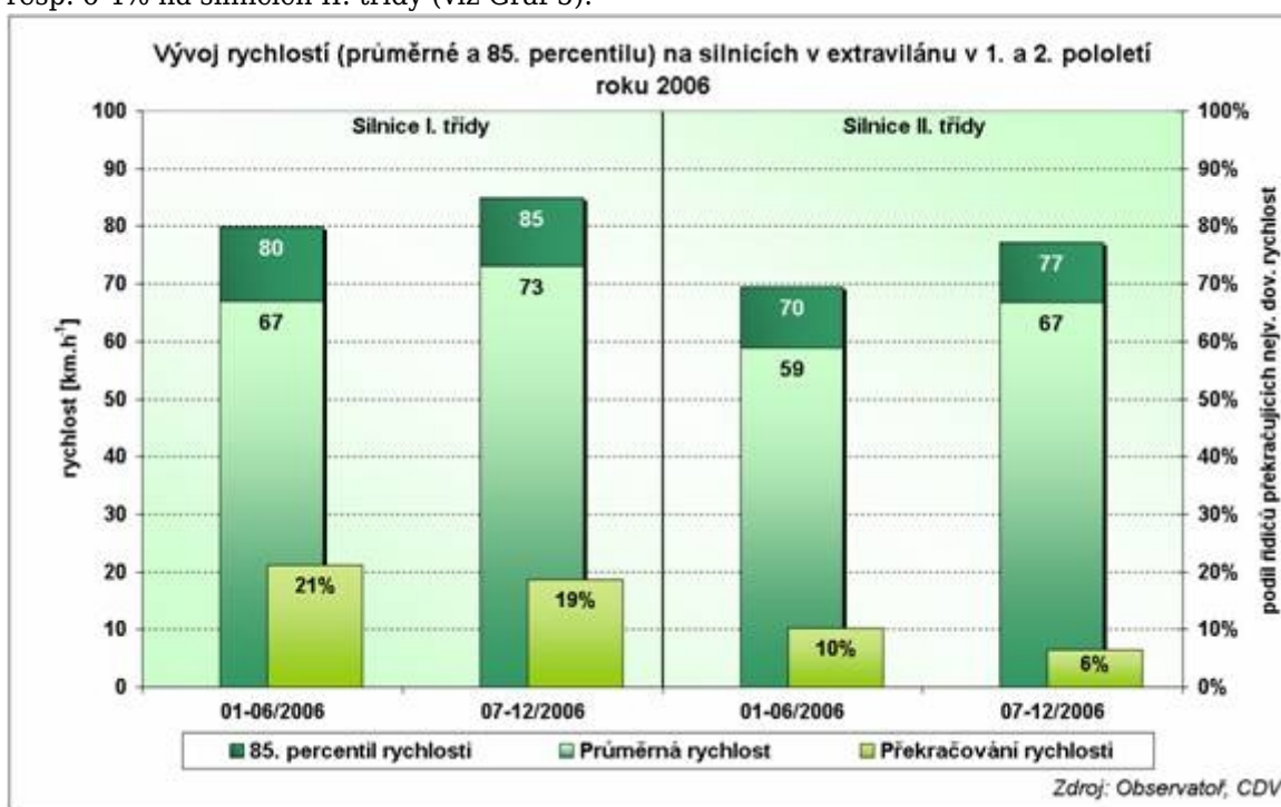
Graf 1: Porovnání rychlostí a překračování nejvyšší dovolené rychlosti na silnicích I. a II. třídy v extravilánu v prvním a druhém pololetí roku 2006
