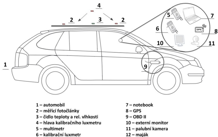
Schéma měřicího vozidla využívající systém MOMOK®
