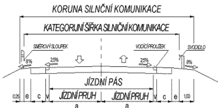
Obr. 1 – příčný řez směřově nedělenou komunikací
