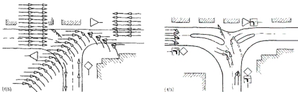
Obr. 16: Příklad srovnání nehodovosti na křižovatce se zalomenou předností bez úprav a s úpravami
