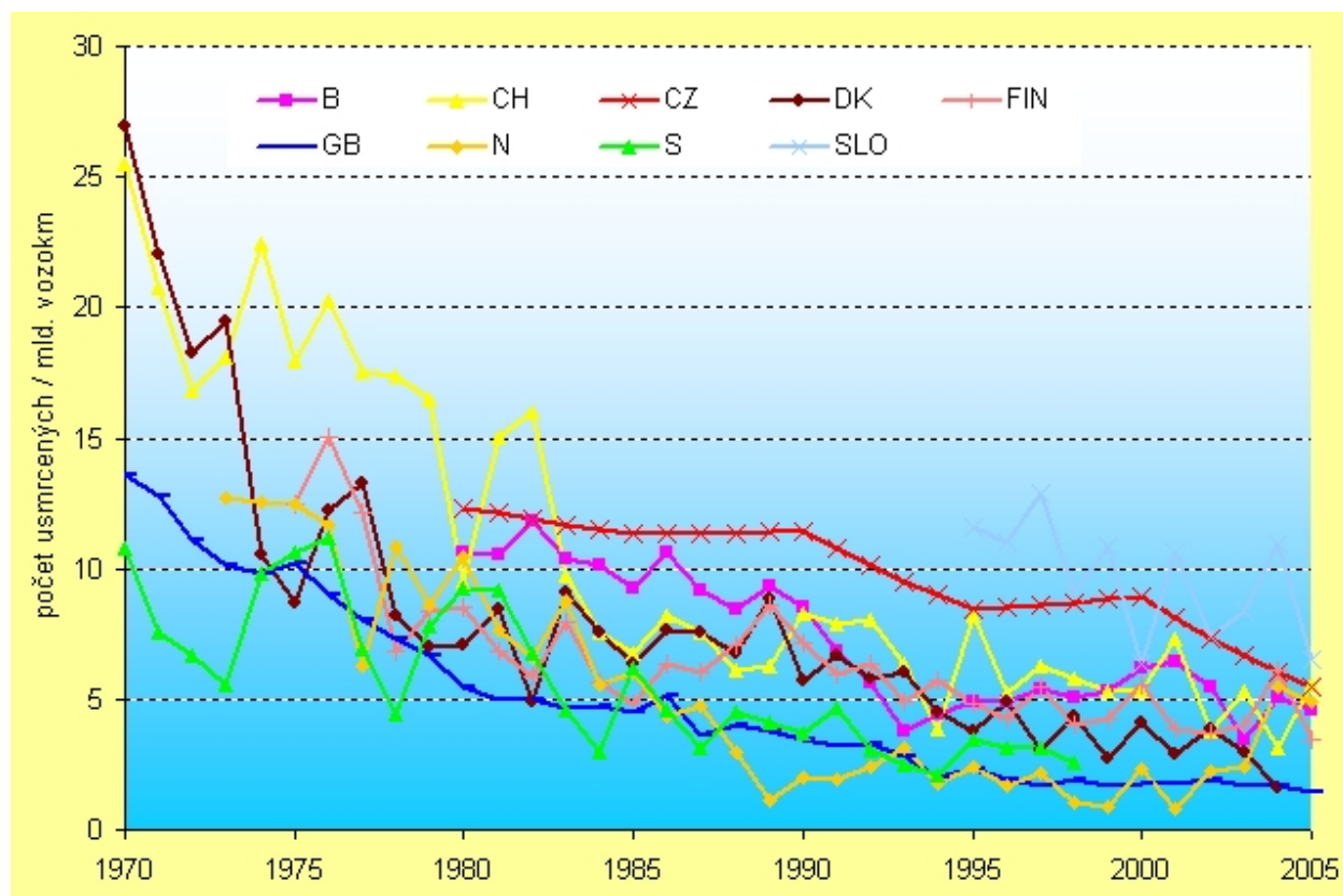
Graf 1: Vývoj míry rizika - počet usmrcených na 1 mld. vozokm pro těžká vozidla (nákladní automobily a autobusy) (1970 - 2005)
