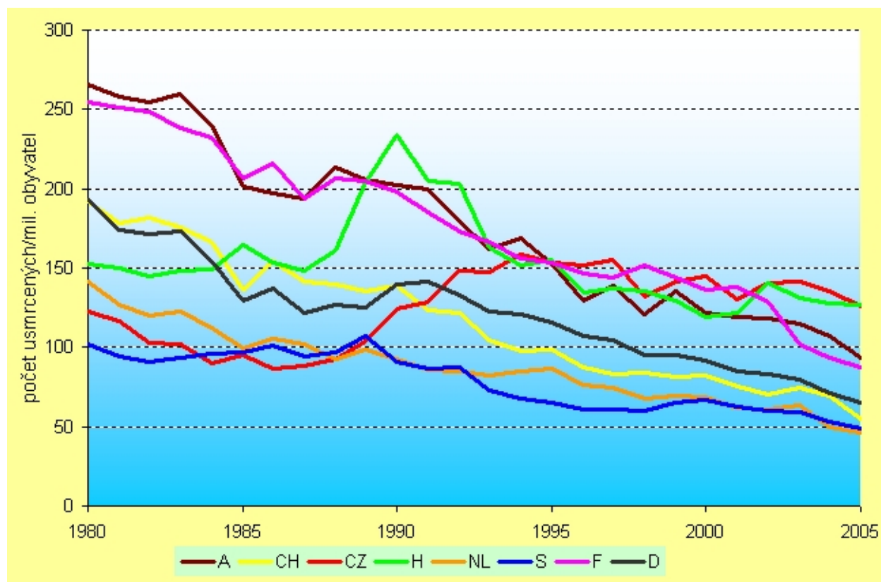
Graf 4: OECD - usmrčení v silničním provozu na mld. vozokm (2005)
