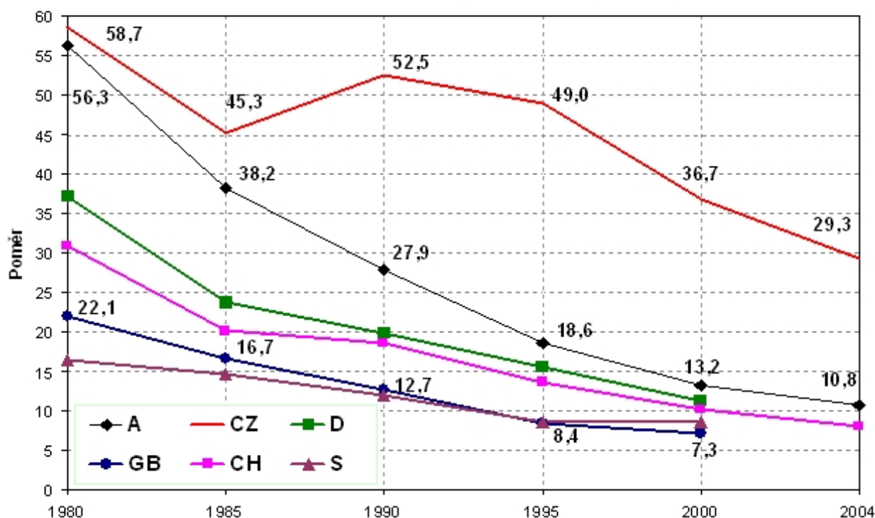
Graf 1c: Usmrčení na PK na 10exp9 vozidlokm (1980 - 2004)
