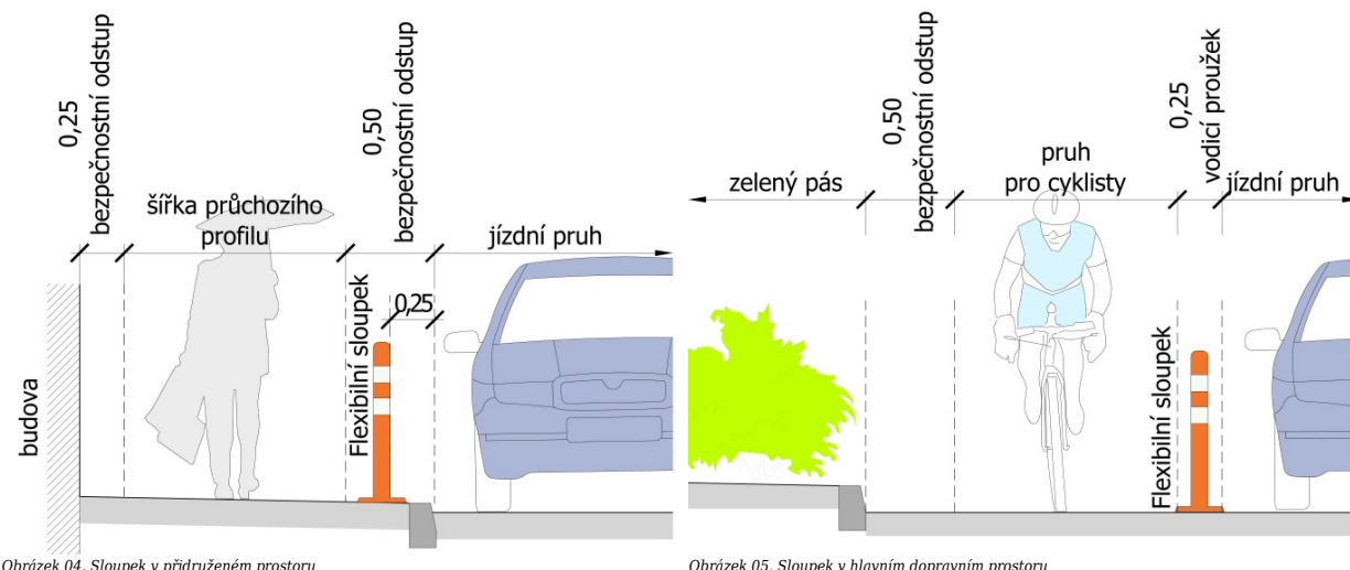
Obrázek 04. Sloupek v předruženém prostoru
