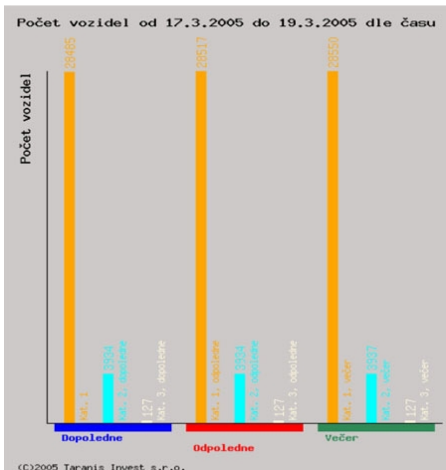
Obr. 3.7.1-1: Editace grafu
