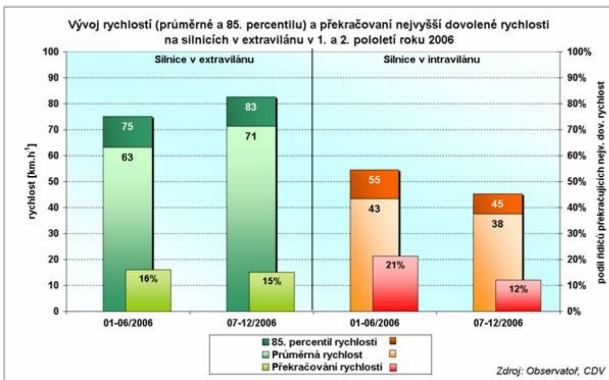
Graf 1: Porovnání rychlostí a překračování nejvyšší dovolené rychlosti v extravilánu a intravilánu v prvním a druhém pololetí roku 2006
