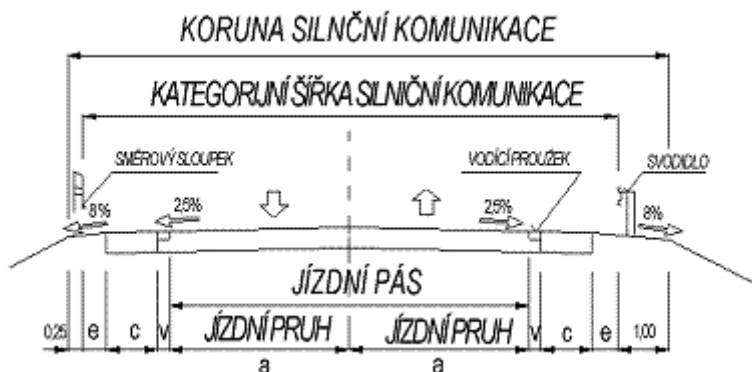
Obr. 1 – příčný řez směrův nedělenou komunikací
