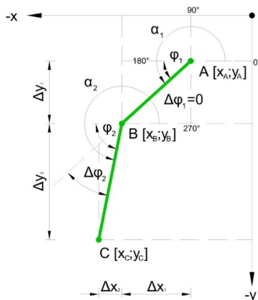
obrázok 05. Základní konstrukce trajektorie pohybu vozidla pro analýzu jeho pohybu (prezentováno na systému S-JTSK)
