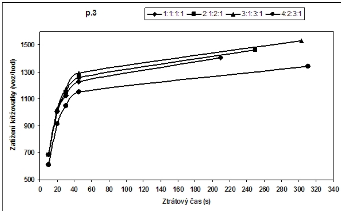
Zátěžové charakteristiky na dispozičním uspořádání p.3
