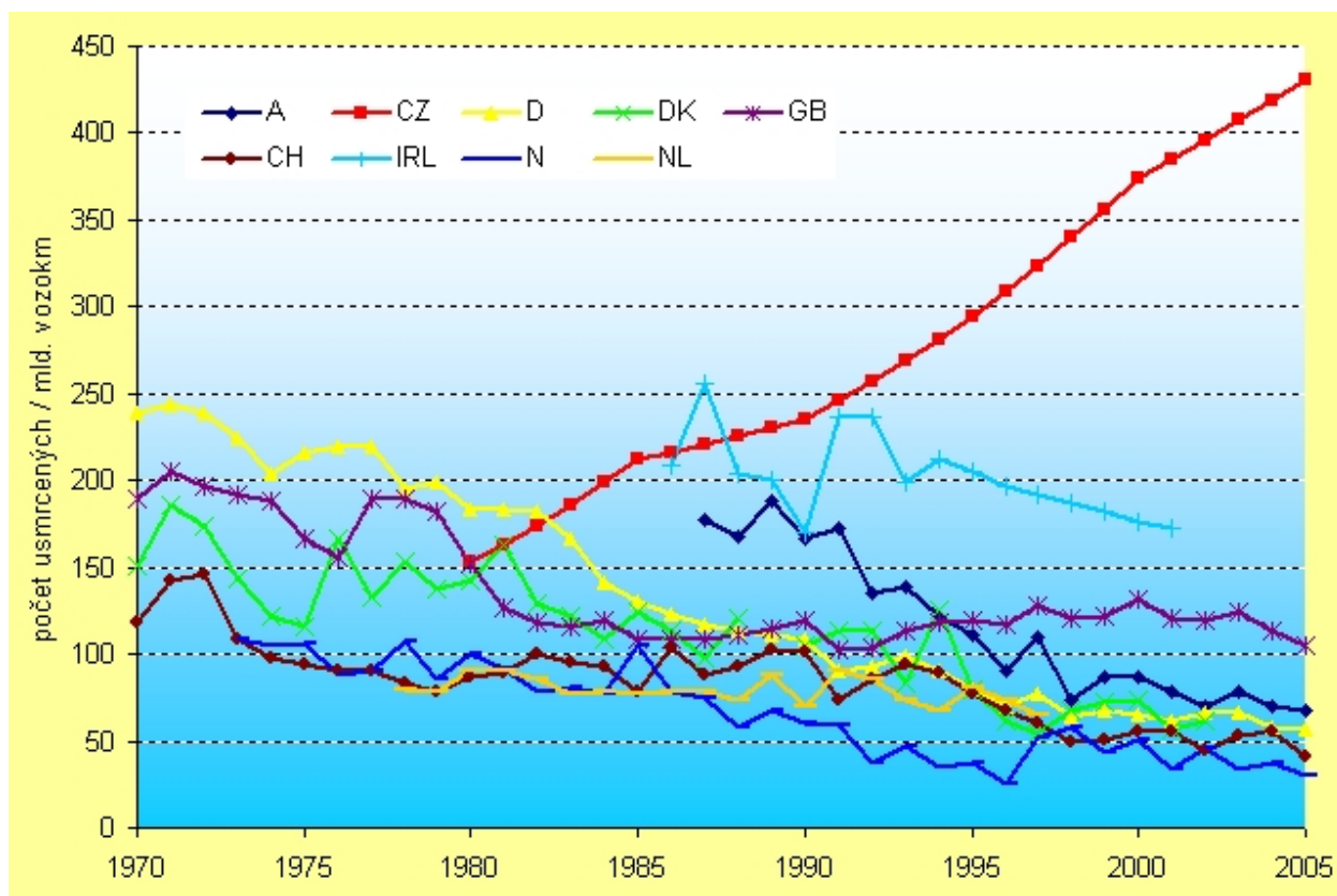
Graf 1: Vývoj míry rizika - počet usmrcených na 1 mld. vozokm pro motocykly a mopedy (1970 - 2005)
