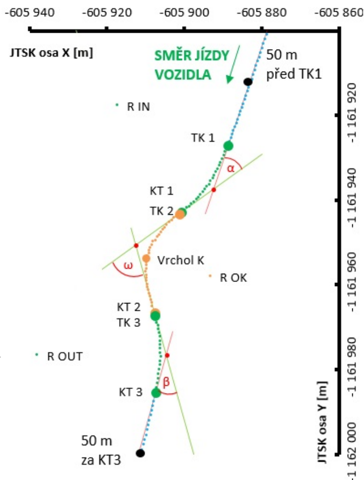
obr. 06.Konstrukce trajektorie přímého průjezdu na OK (skutečný průjezd)
