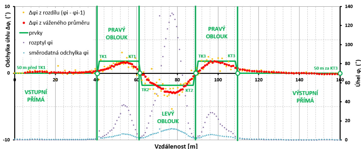
obr. 07. Identifikace prvků trajektorie pomocí směrových úhlů \varphi_i a jejich odchylek \Delta\varphi_i
