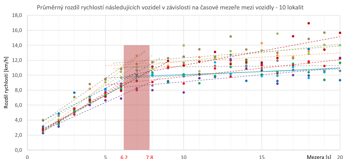
obr. 02. Pražová hodnota ovlivnění řidičů dle průměrného rozdílu rychlosti po sobě jedoucích vozidel
