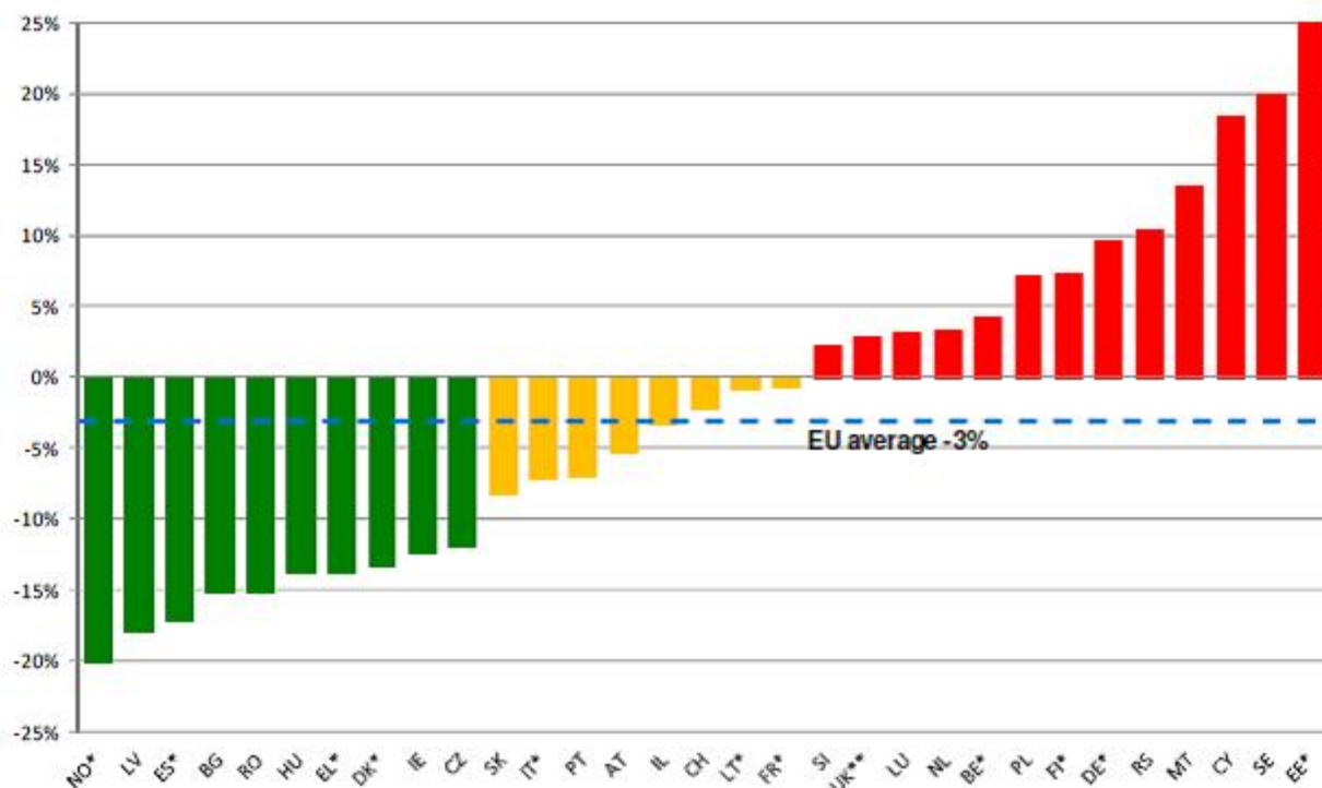
Graf 2 - Počet usmrcených vztažený na miliardu ujetých vozokilometrů (průměr pro poslední 3 roky dostupných dat)
