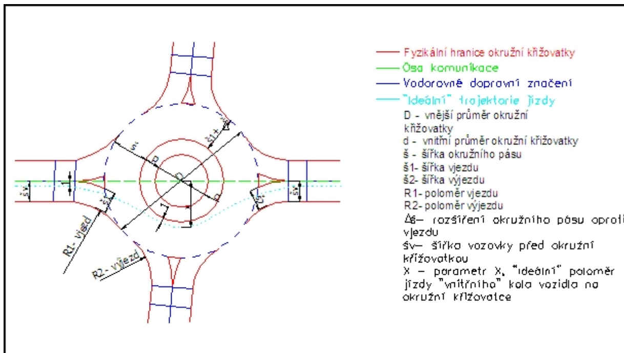
Označení parametrů pro soubor okružních křižovatek - Geometrie
