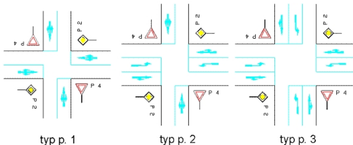
Dispoziční uspořádání typů průsečných křižovatek
