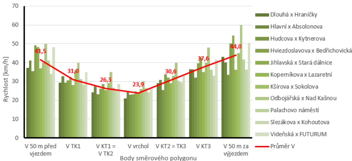
obr. 08. Rychlost měřicího vozidla na přímém průjezdu OK v bodech směrového polygonu
