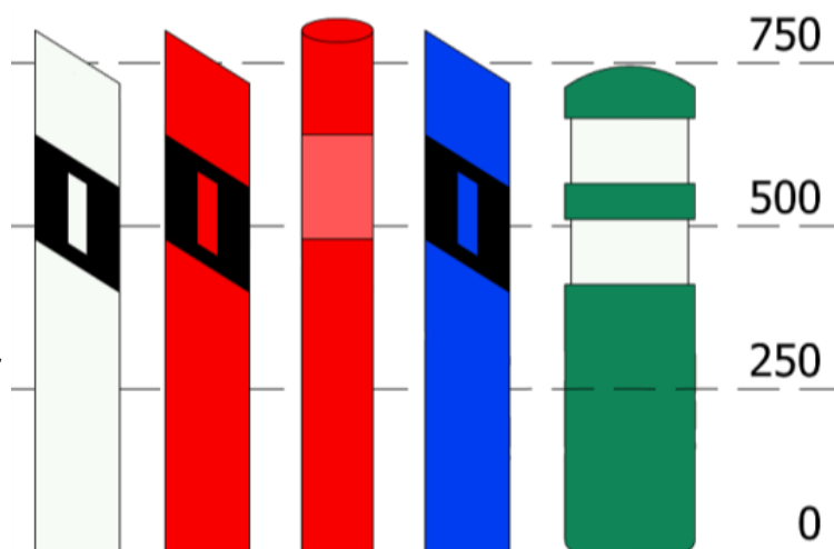
Obrázek 01. Směrové sloupky
