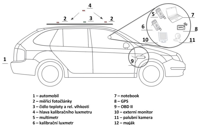
Schéma měřicího vozidla využívající systém MOMOK®
