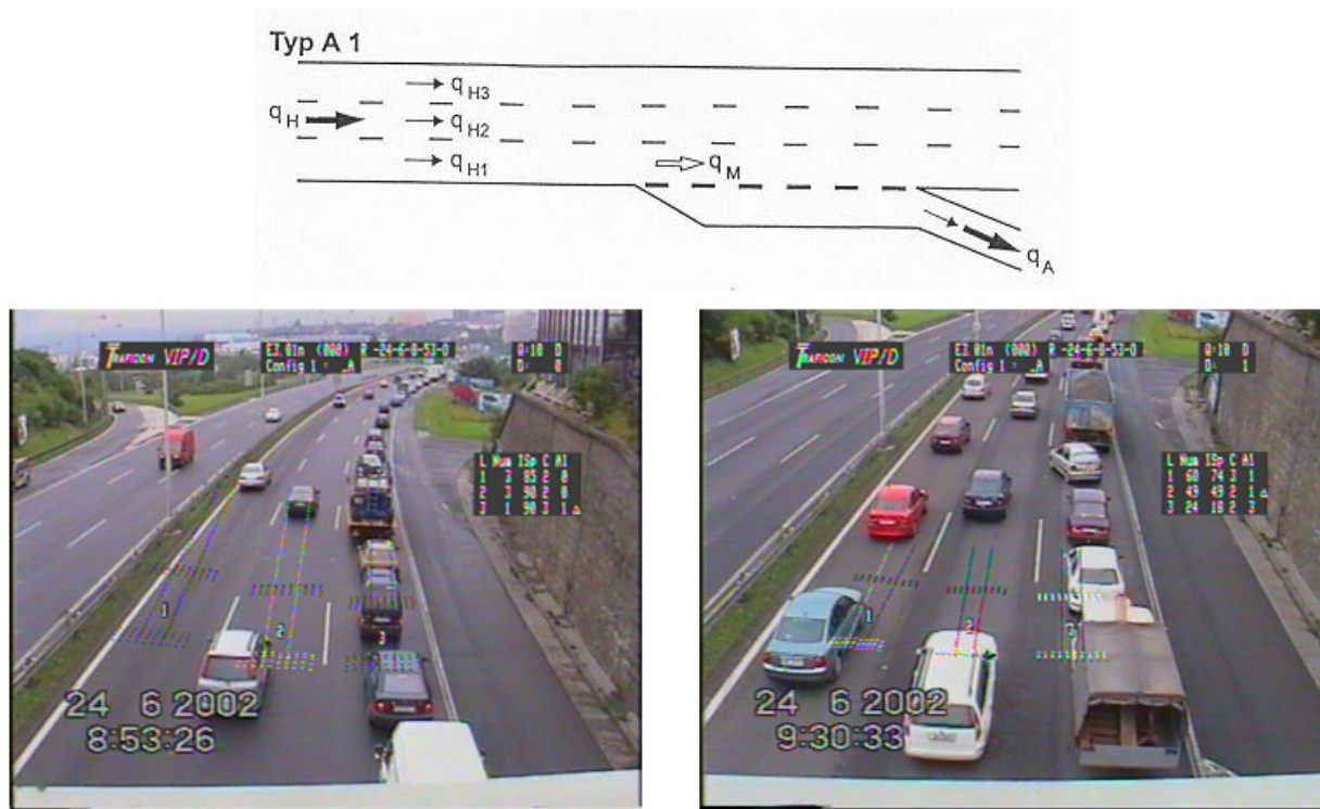
Obr. 5 Schéma a základní reálný videoobraz sledovaného odbočování
