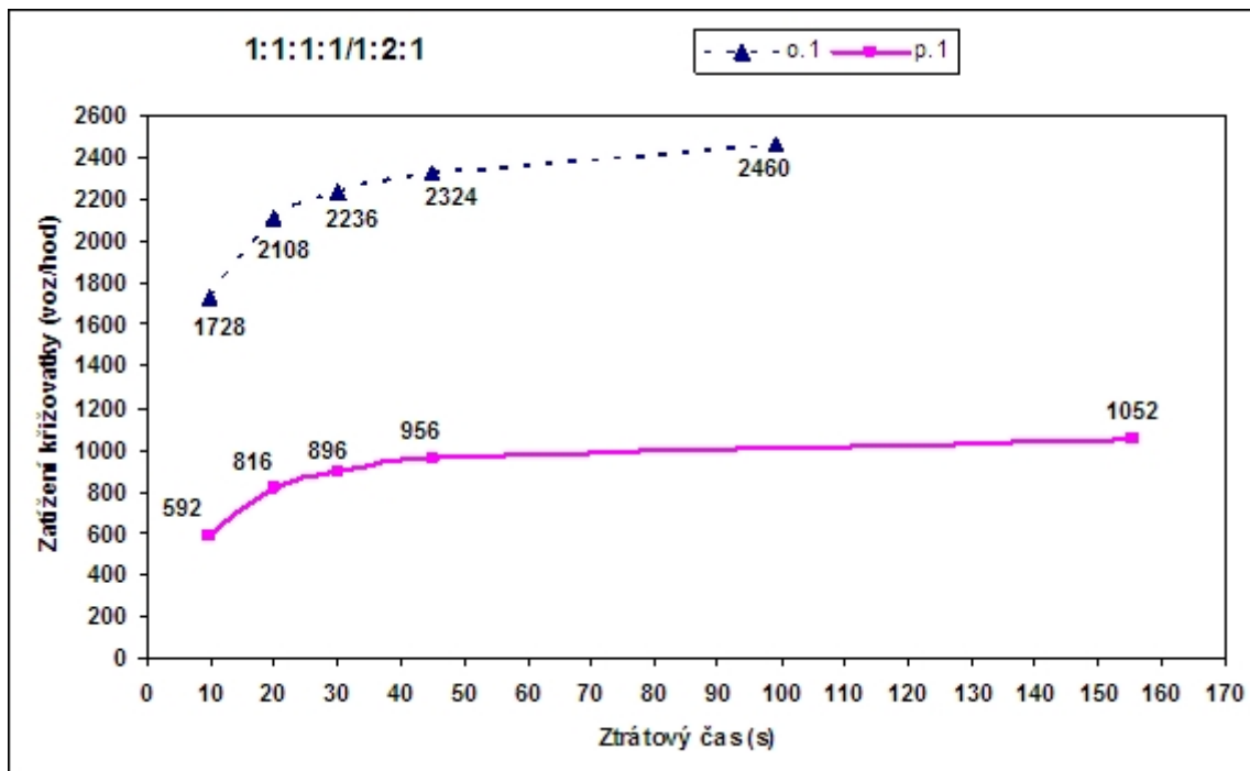
Porovnání celkového zatížení křižovek v závislosti na ztrátovém čase
